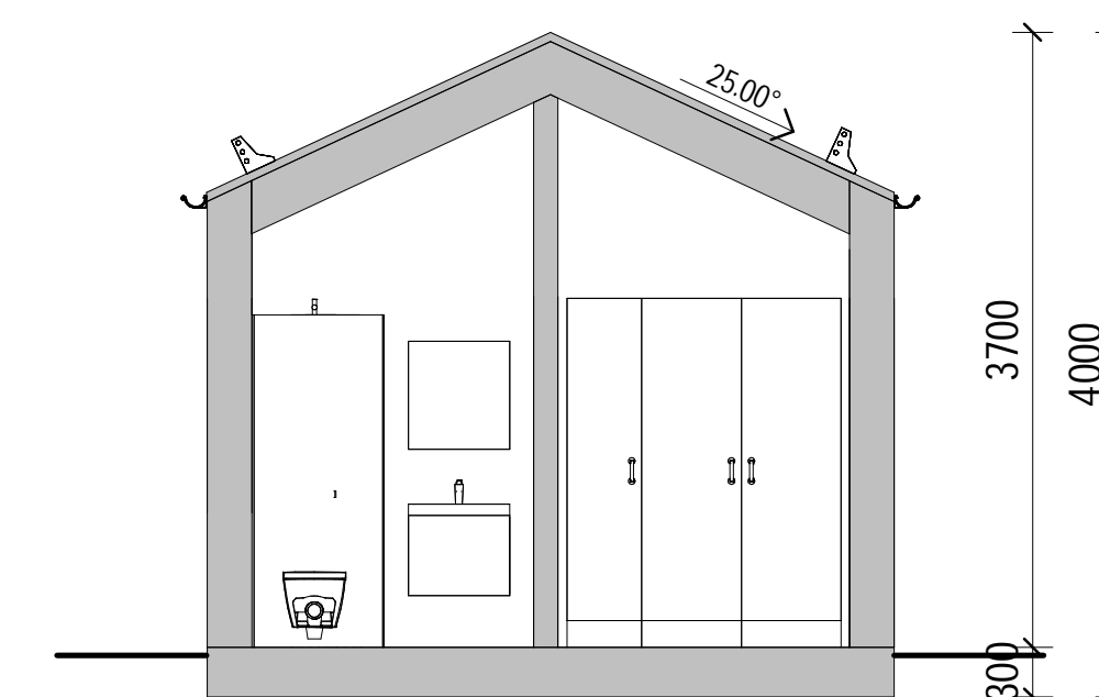
SEKTION A-A
